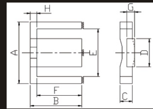
FIG(2) EFD-A
