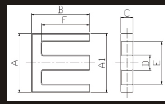
FIG(3) EFD-A
